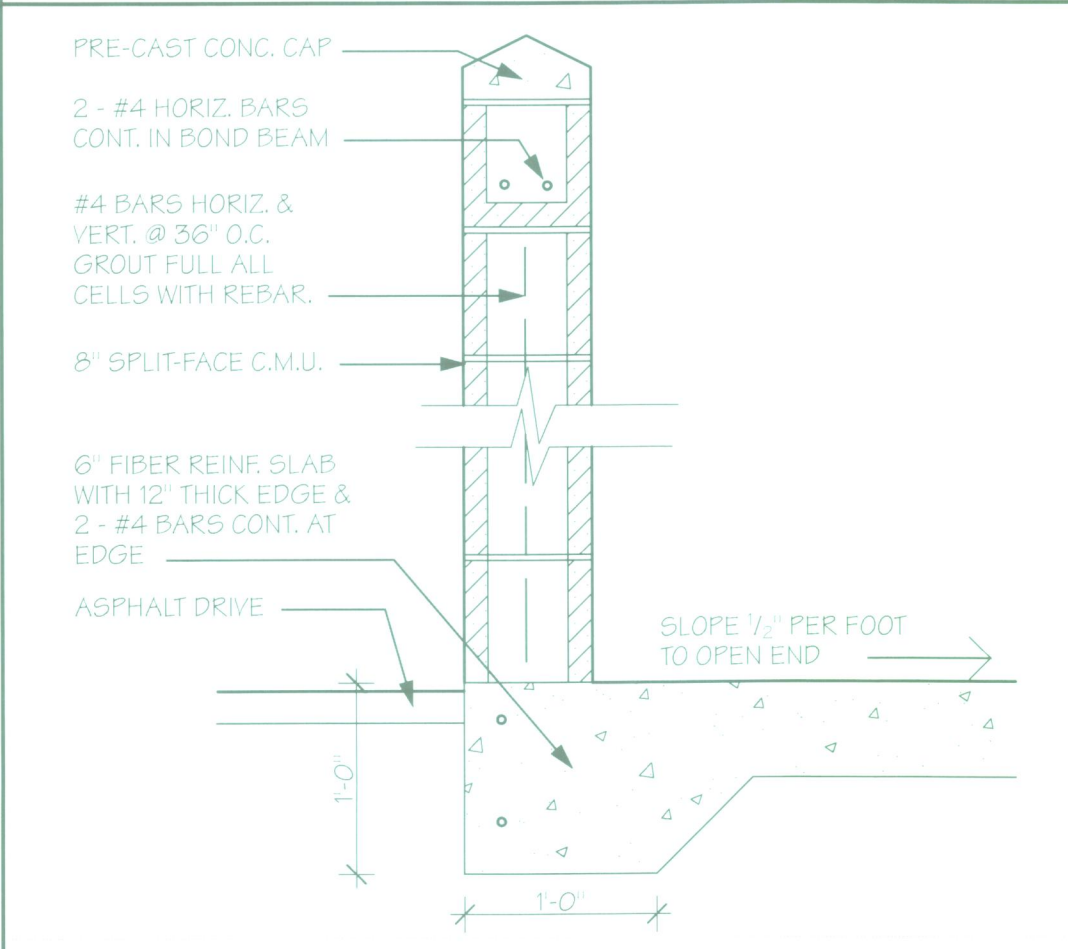
4 TRASH ENCLOSURE SECTION SCALE: 1" = 1'-0"
