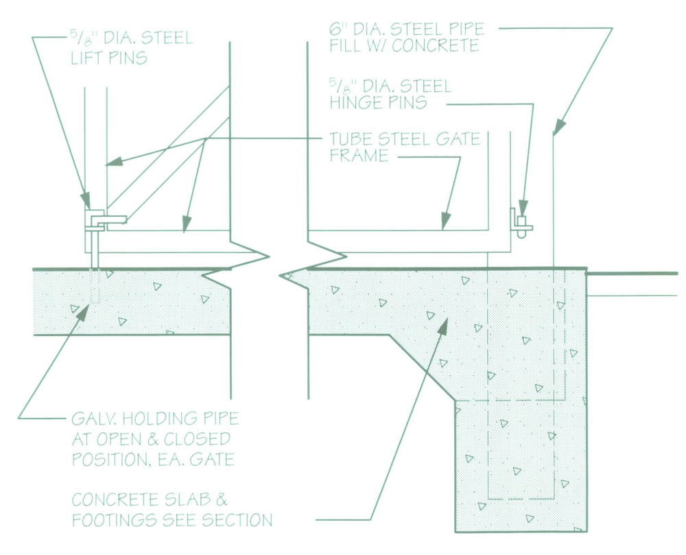
5 TRASH GATE SECTION SCALE: 1" = 1'-0"
