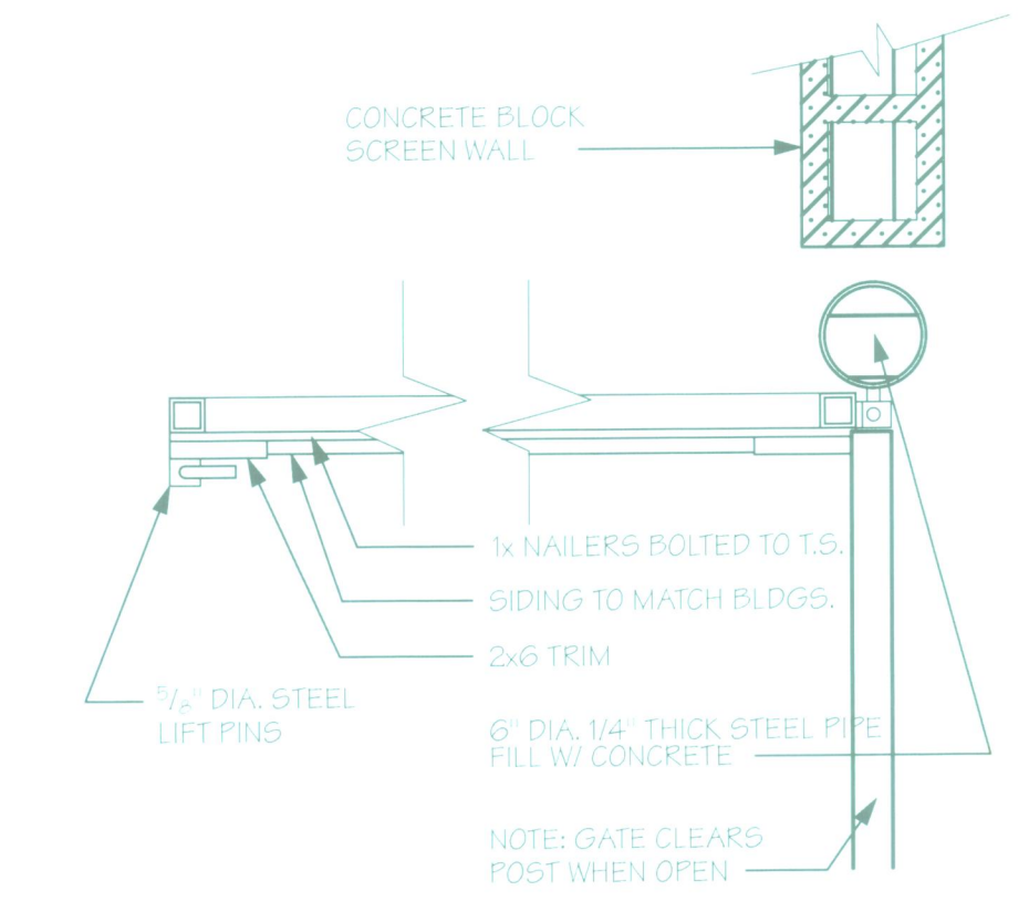
6 TRASH GATE PLAN SCALE: 1" = 1'-0"
